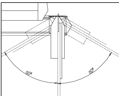
Toute la table peut tourner de -60° jusqu'à +60°.
