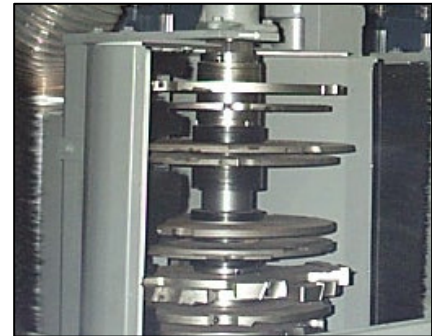
Plusieurs jeux d'outils peuvent être montés sur les arbres longs de 545.
