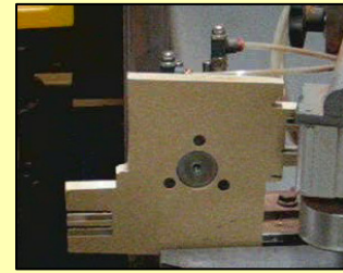
Pare-éclats pneum. avec 2 positions automatiques
