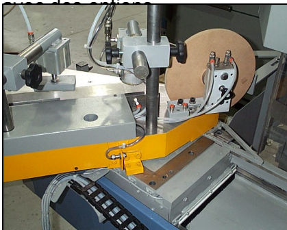
Toute la table peut tourner de -60° jusqu'à +60°.
